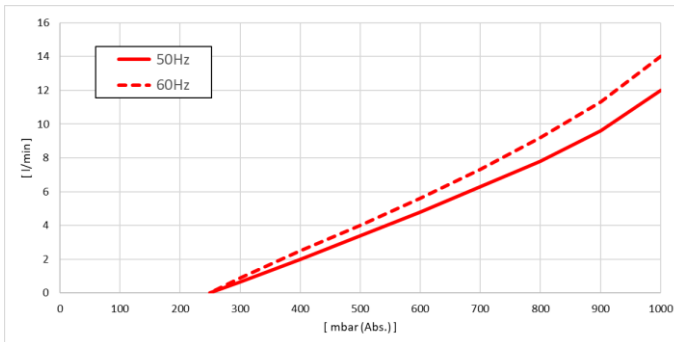
NOTA: Curve riferite alla pressione di 1013mbar (ass.) e temp. 20°C (tolleranza ±10%).
